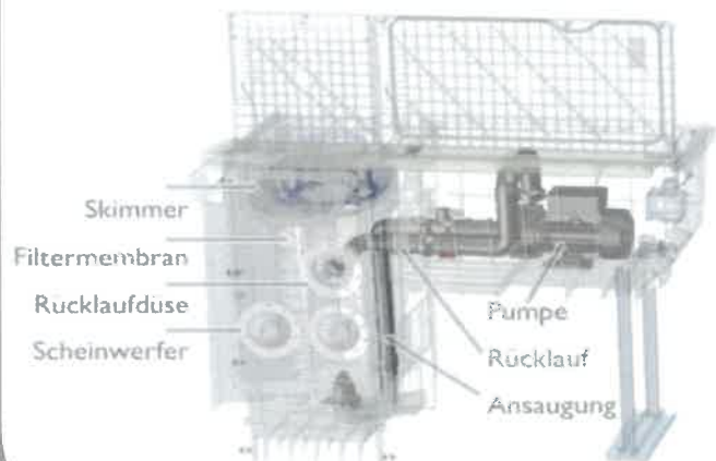
Beispiel-Schema Filter
